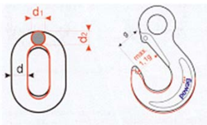
Dimensionsprüfung
