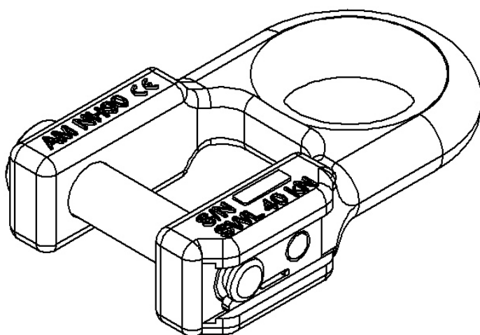
Fig.: Accessorio per imbracatura P/N AM_NH90, certificato secondo EN 1677-A1 (misura 13), da utilizzare con elicotteri NH90 (Annex I) Progettazione: A&H Engineering, Design Felix Muheim Formenbau Altdorf, Schmiedewerk pewag austria
