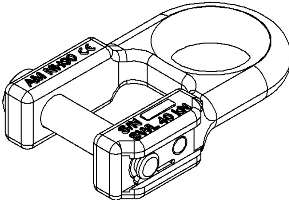
Abb.: Anschlagmittel P/N AM_NH90, qualifiziert nach EN 1677-A1 (Grösse 13), im Einsatz mit NH90 (Annex II) Entwicklung A&H ENG, Design Felix Muheim Formenbau Altdorf, Schiedewerk pewag austria
